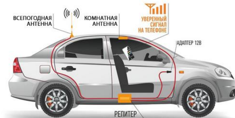
Схема №1. Пример мест установки оборудования для усиления сотового сигнала
